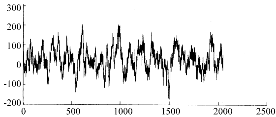
Fig. 2: Noisy EEG
