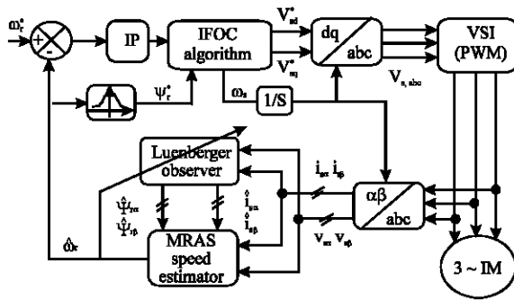
Fig. 4: Sensorless IFOC scheme of IM
