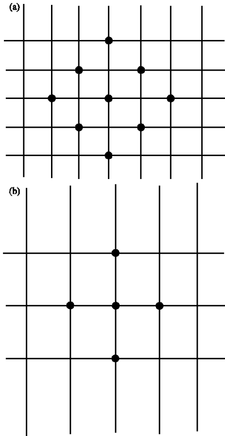
Fig. 2: Diamond search pattern a) LDSP; b) SDSP
