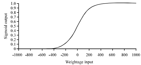
Fig. 3: Sigmoid function
