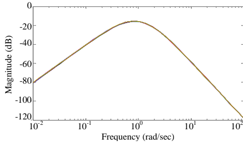
Fig. 8: GP-G_{norm}
