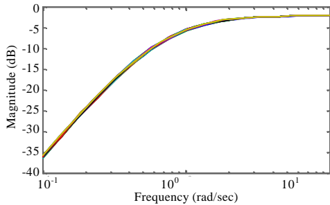
Fig. 10: G_p-G_{norm}/G_{norm}
