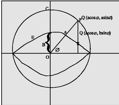
Fig. 4: Parametric circle
