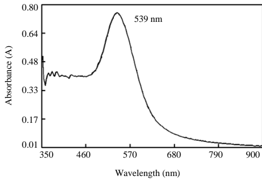
Fig. 5: UV-visible spectrum of gold nanoparticles (D)
