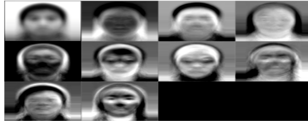
Eigenfaces
